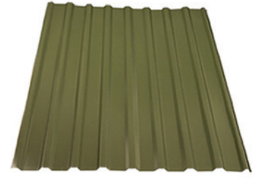
Profilipelti JTE-20 Hyötyleveys 1090 mm
